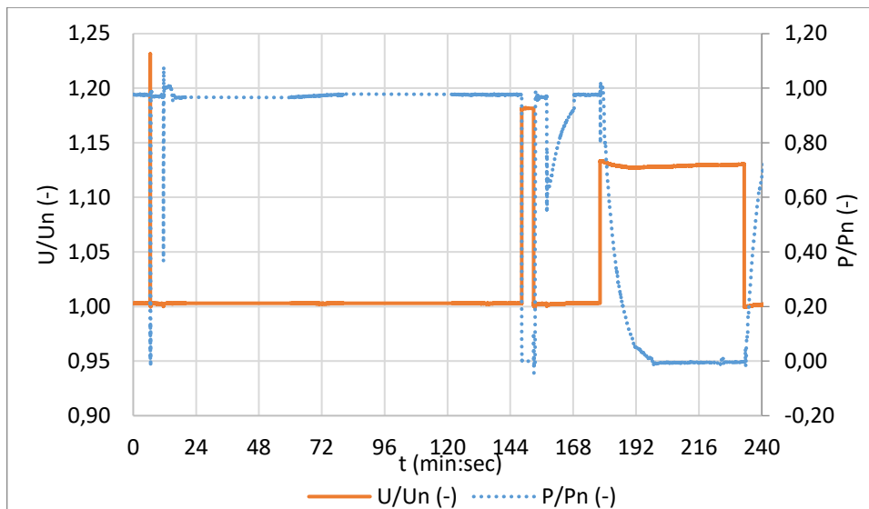
Obr.10.2: Křivka ORVT
