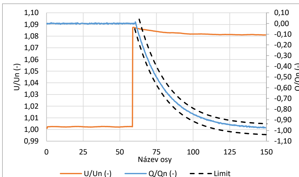
Obr.11.5: Dynamická odezva jalového výkonu Q na skokovou změnu napětí U
