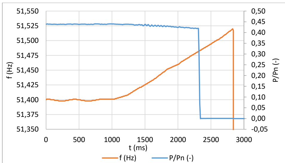
Obr.12.9: Nadvýkennční ochrana
