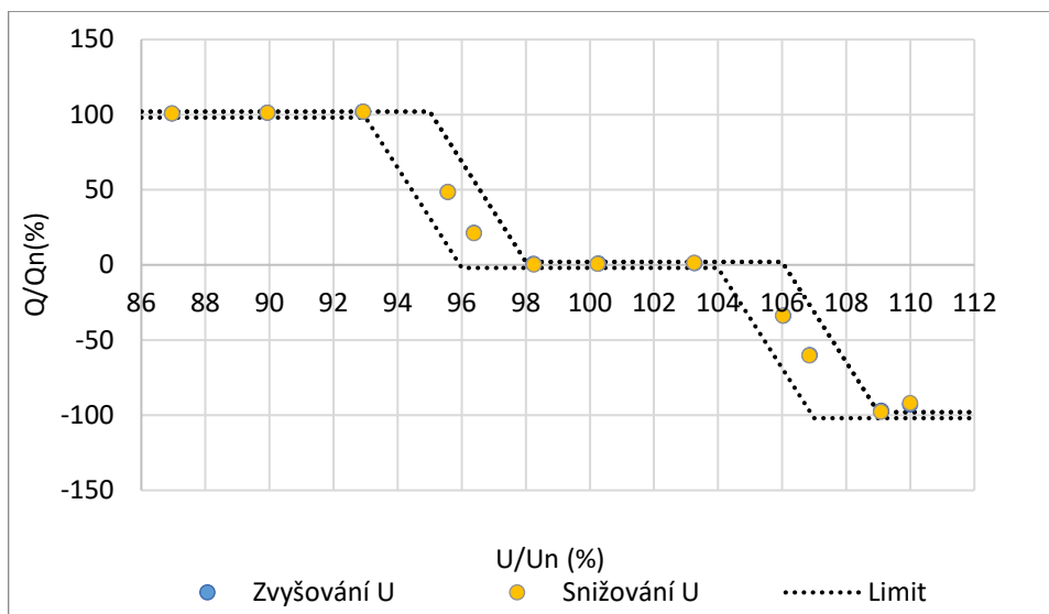
Obr.11.4: Q(U) – vyhodnocení
