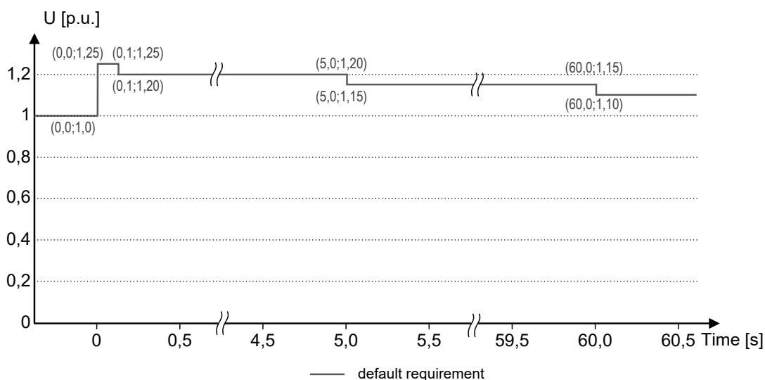
Obr.10.1: Křivka ORVT
