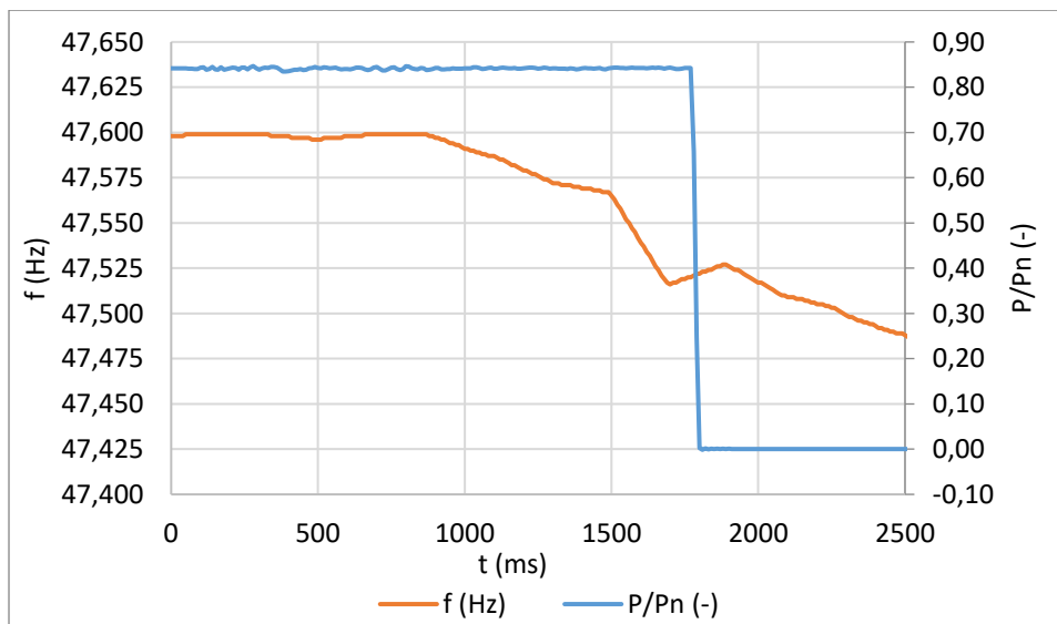
Obr.12.10: Podvýkennční ochrana
