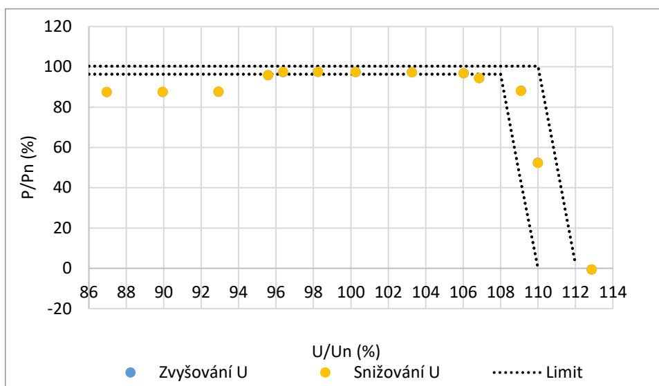
Obr.11.2: P(U) – vyhodnocení
